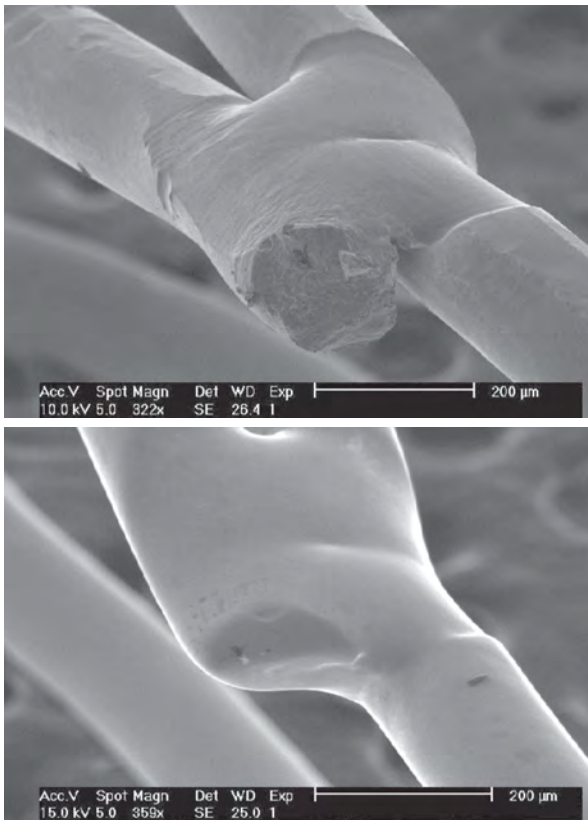
Figura 12. Îmbinarea sudată a stentului TentaFlex înainte și după lustruirea electrochimică / Figure 12. Welded joint of the TentaFlex stent before and after electropolishing
