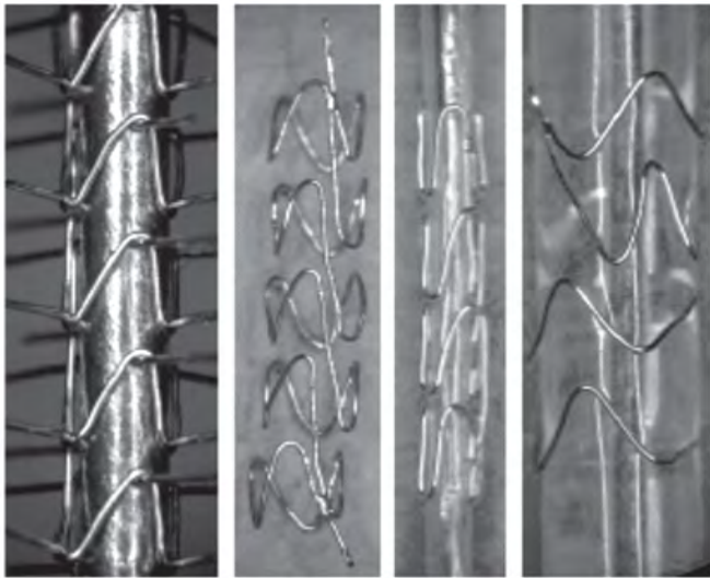
Figura 11. Producerea și pașii expansiunii balonului / Figure 11. Producing and balloon expansion steps
