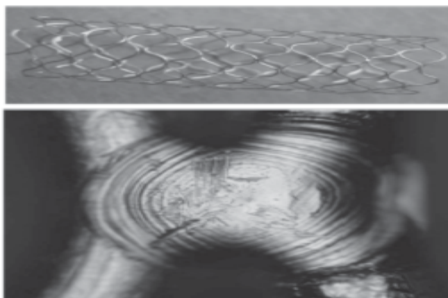
Figura 8. Prototipul stentului ultra-flexibil sudat cu laser (suprafața netratată) / Figure 8. Prototype of laser welded ultra-flexible stent (untreated surface)
